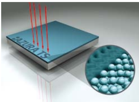
Belichtete :Azura TS-Druckplatte Die Emulsion absorbiert die Energie des mit einer Wellenlänge von 830 nm arbeitenden Lasers. Die ThermoFuse™-Partikel verschmelzen miteinander und gehen eine feste Verbindung mit dem aufgerauten und anodisierten Aluminiumschichtträger ein.
